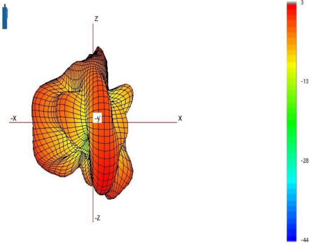
(6) 2500MHz 的 3D 方向图:
