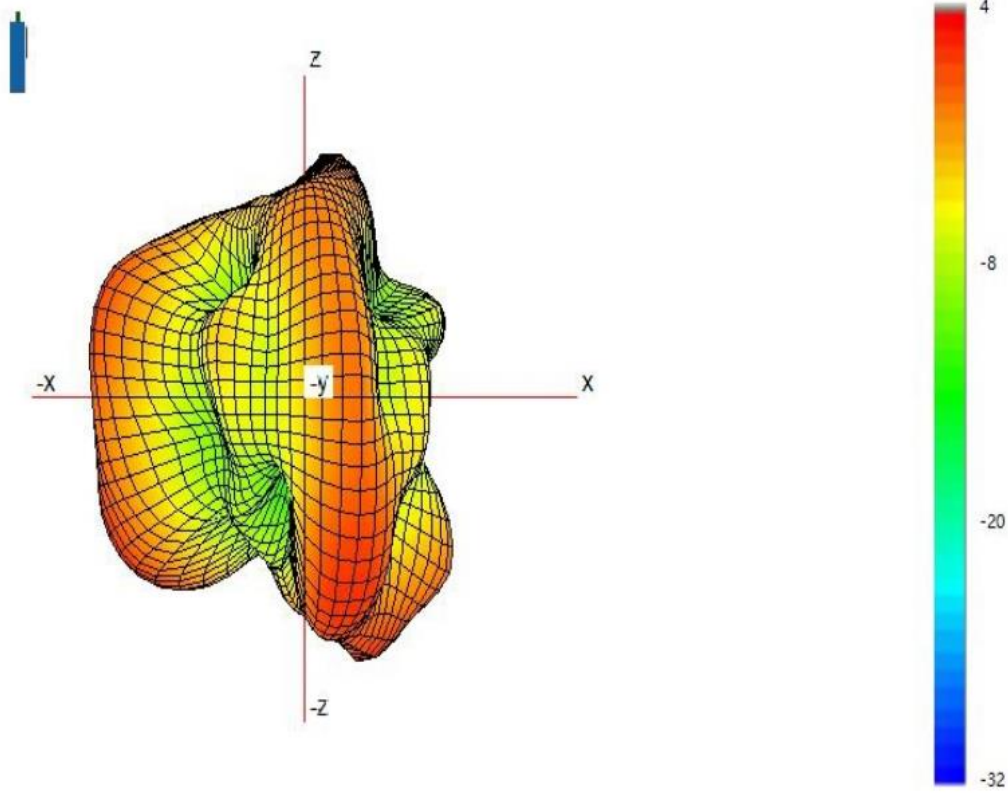
(5) 2442MHz 的 3D 方向图:
