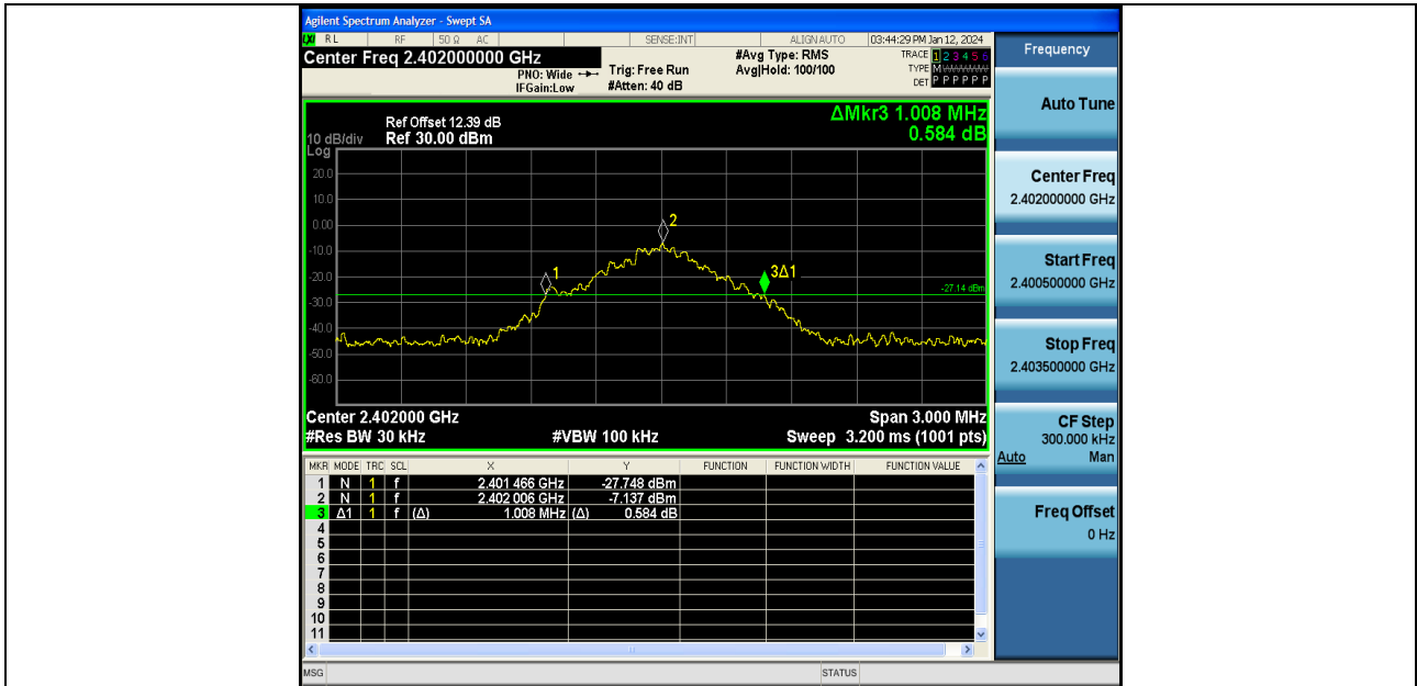
DH5-Ant1-2402
