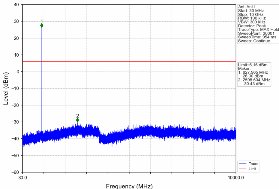
50kbps_HOPP_Ant1_NTNV
