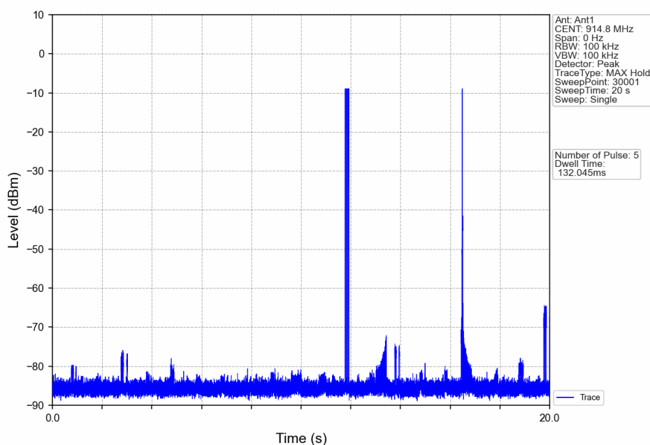
150kbpd_HOPP_Ant1_NTNV
