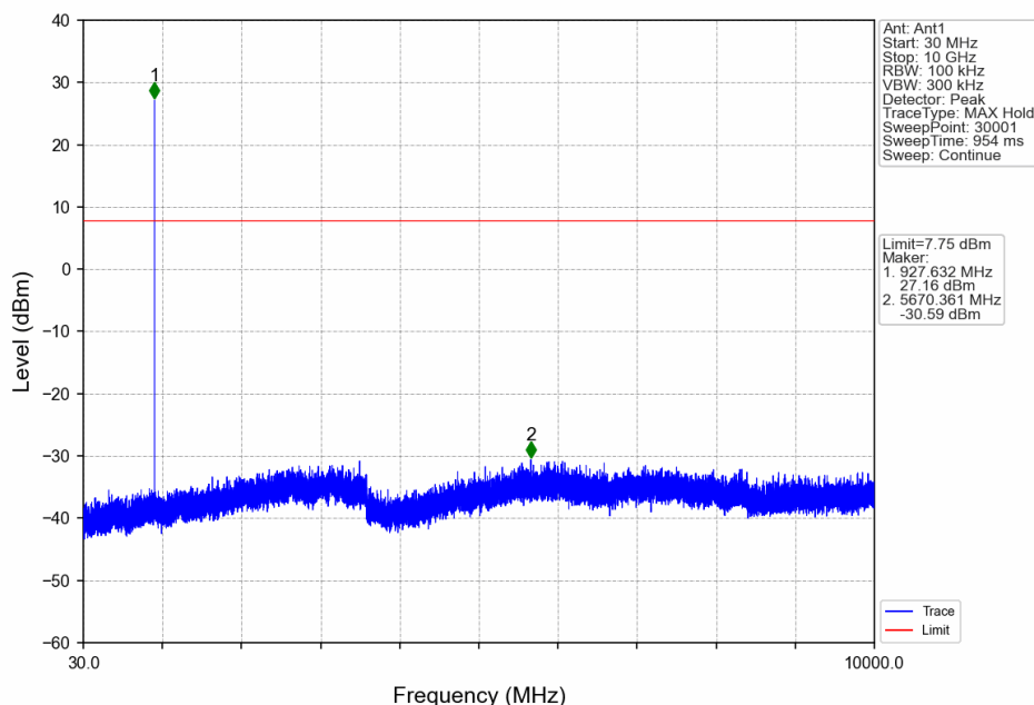
50kbpd_HOPP_Ant1_NTNV
