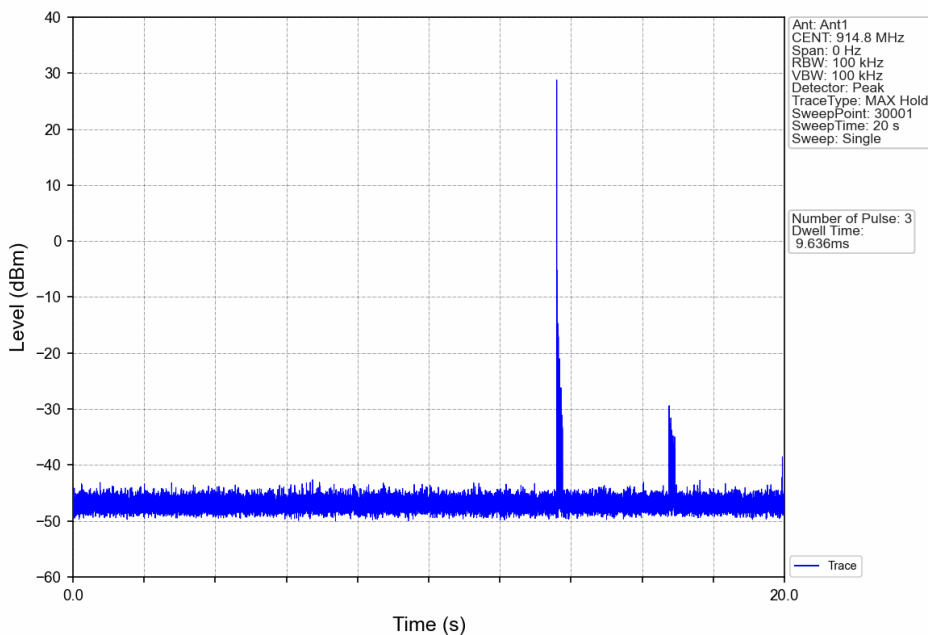
150kbps_HOPP_Ant1_NTNV
