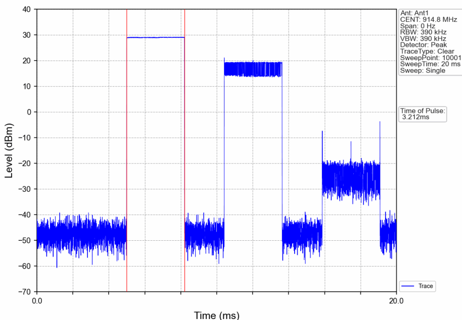
150kbps_HOPP_Ant1_NTNV
