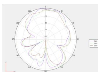
Phi 90 2D 图
