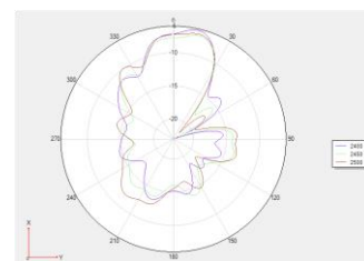
Theta 90 2D 图
