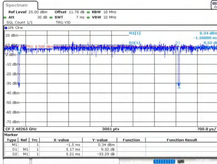
11AX20MIMO_Ant1_2412_26Tone_RU0
