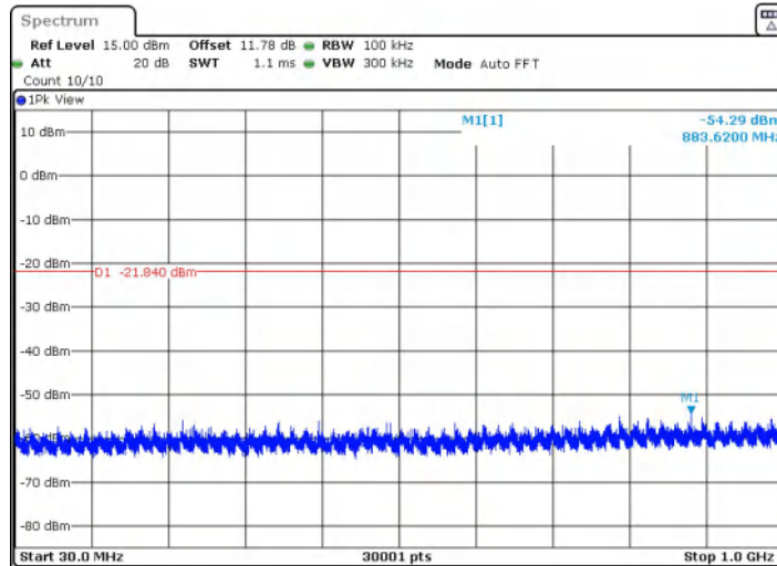
11AX20MIMO_Ant1_2412_26Tone_RU0_30~1000
