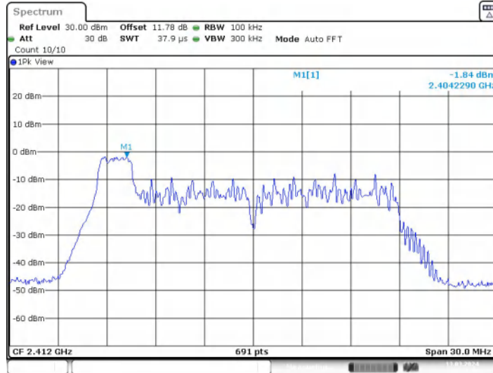
11AX20MIMO_Ant1_2412_26Tone_RU0_0~Reference
