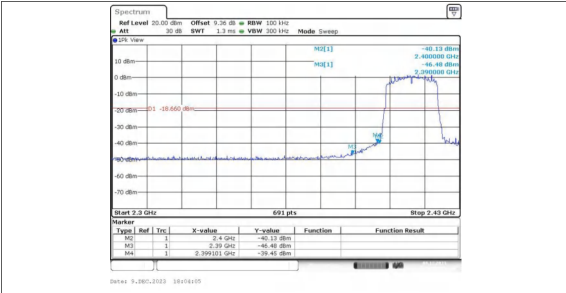
11AX20MIMO_Ant2_Low_2412
