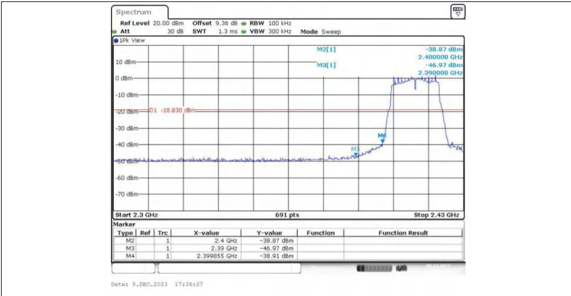
11N20MIMO_Ant2_Low_2412
