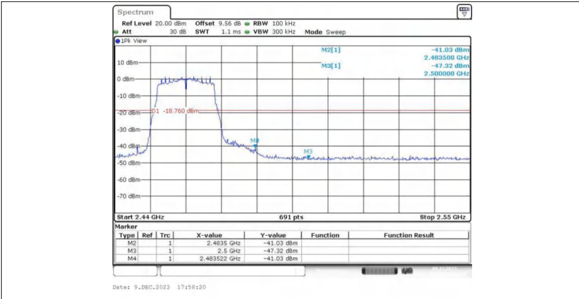
11N20MIMO_Ant2_High_2462
