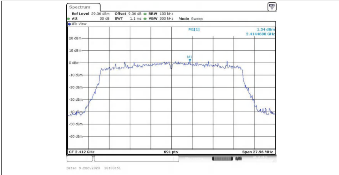
11AX20MIMO_Ant2_2412
