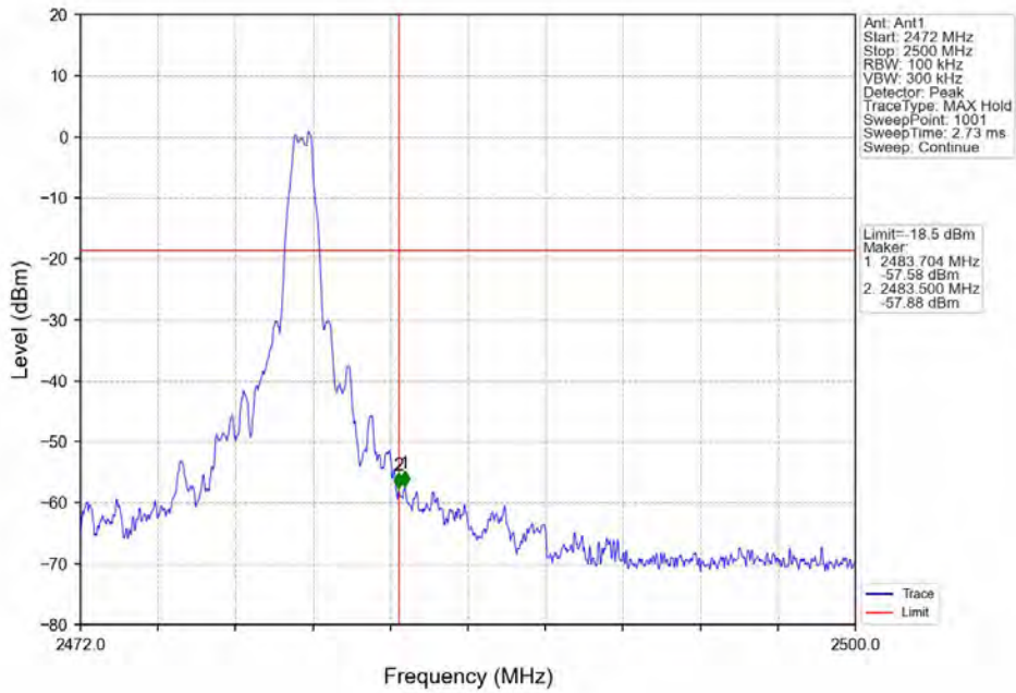
PI/4-QDPSK_HCH_2480MHz_Ant1_NTNV
