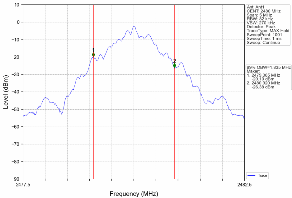
1_HCH_2480MHz_Ant1_NTNV
