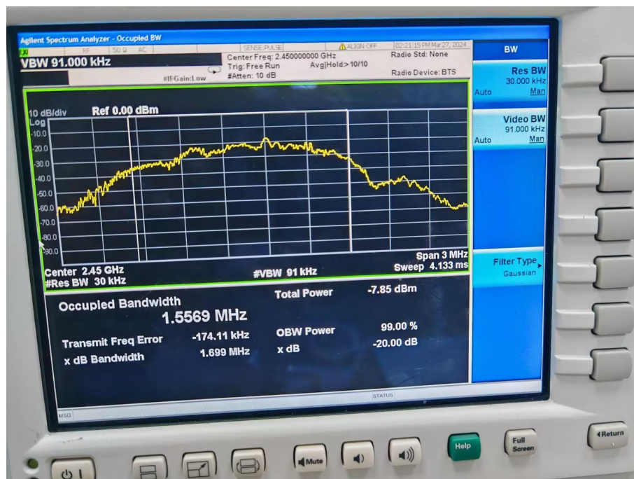
-20dB Bandwidth 2450MHz Ant1
