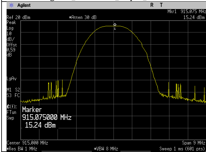
Mid Ch_915MHz_Ouput_Power
