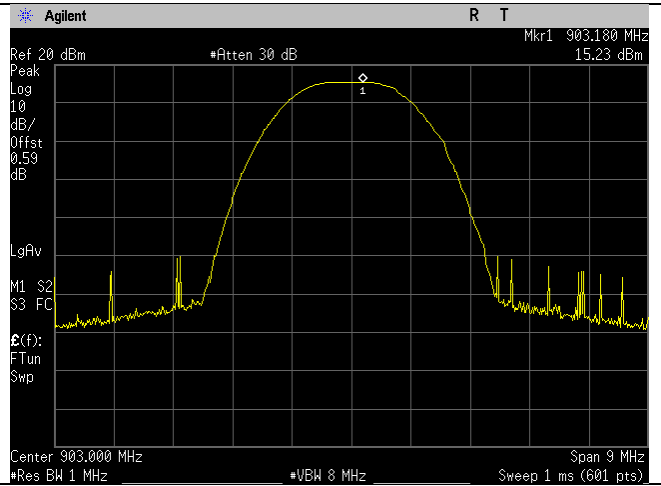
Low Ch_903MHz_Ouput_Power
