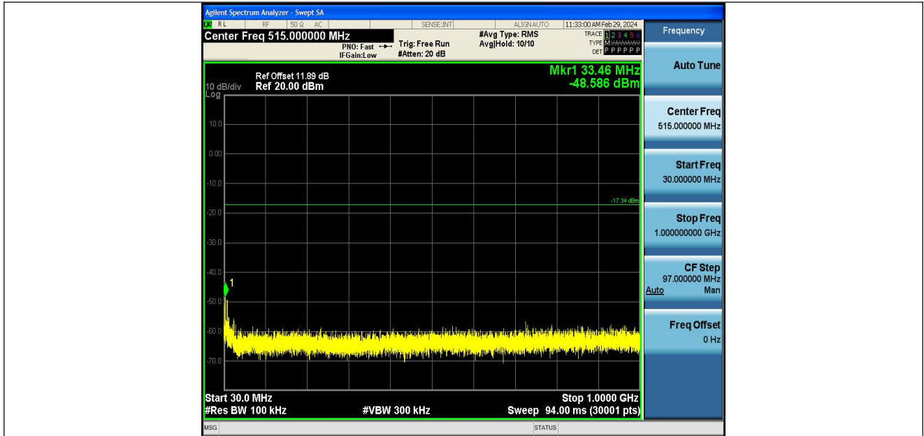
BLE_2M-Ant1-2402-30~1000-PASS
