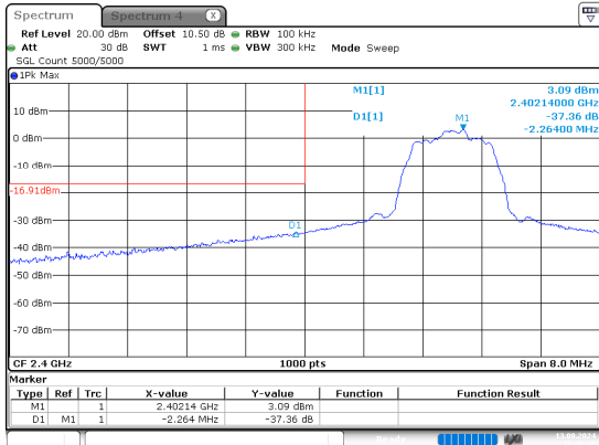
\pi/4 -DQPSK_Low
