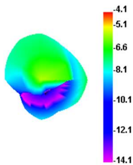
2400.000MHz
