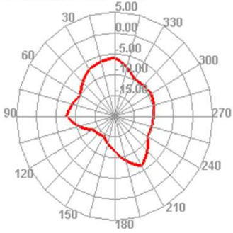
2440.000MHz
