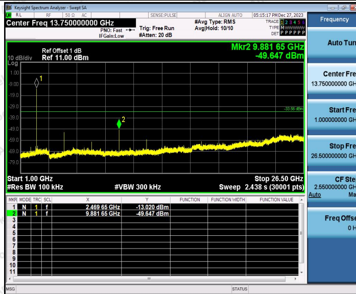
2.4G_Ant1_2470_1000~26500
