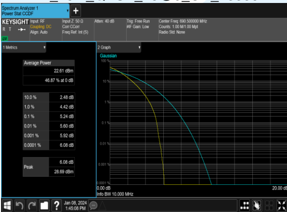
B71_10M_QPSK_50@0_CH_133172
