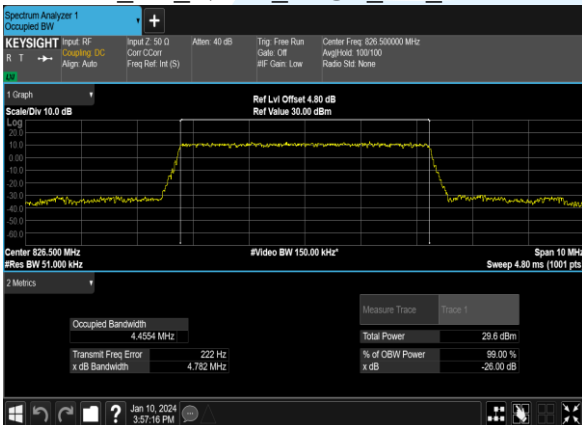
B26_5M_QPSK_25@0_CH_26815
