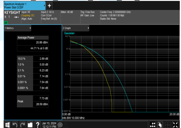
B7_10M_16QAM_50@0_CH_20800
