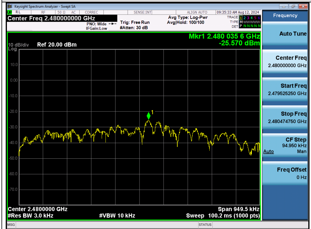
Test_Graph_2.4G_ANT1_2480_PSD
