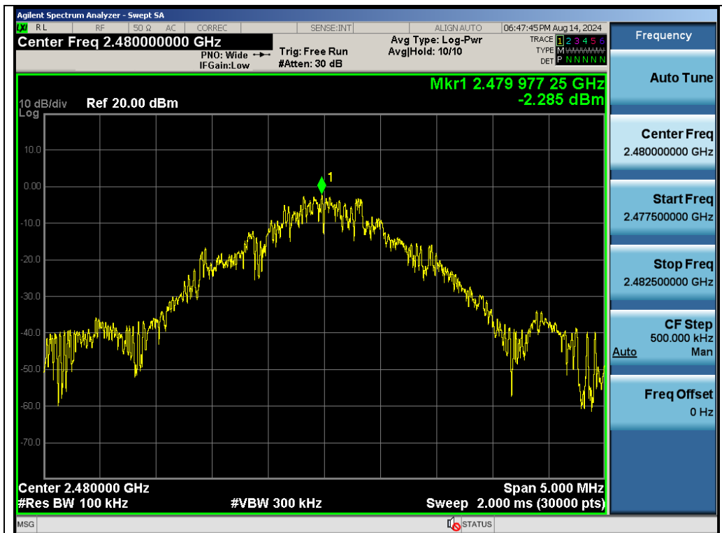
Test_Graph_2.4G_ANT1_2480_Reference Level
