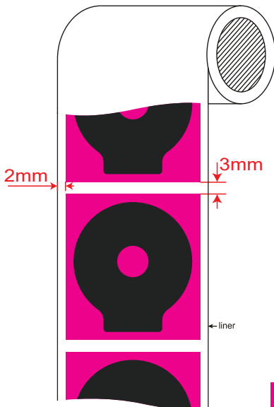
模切示意图
