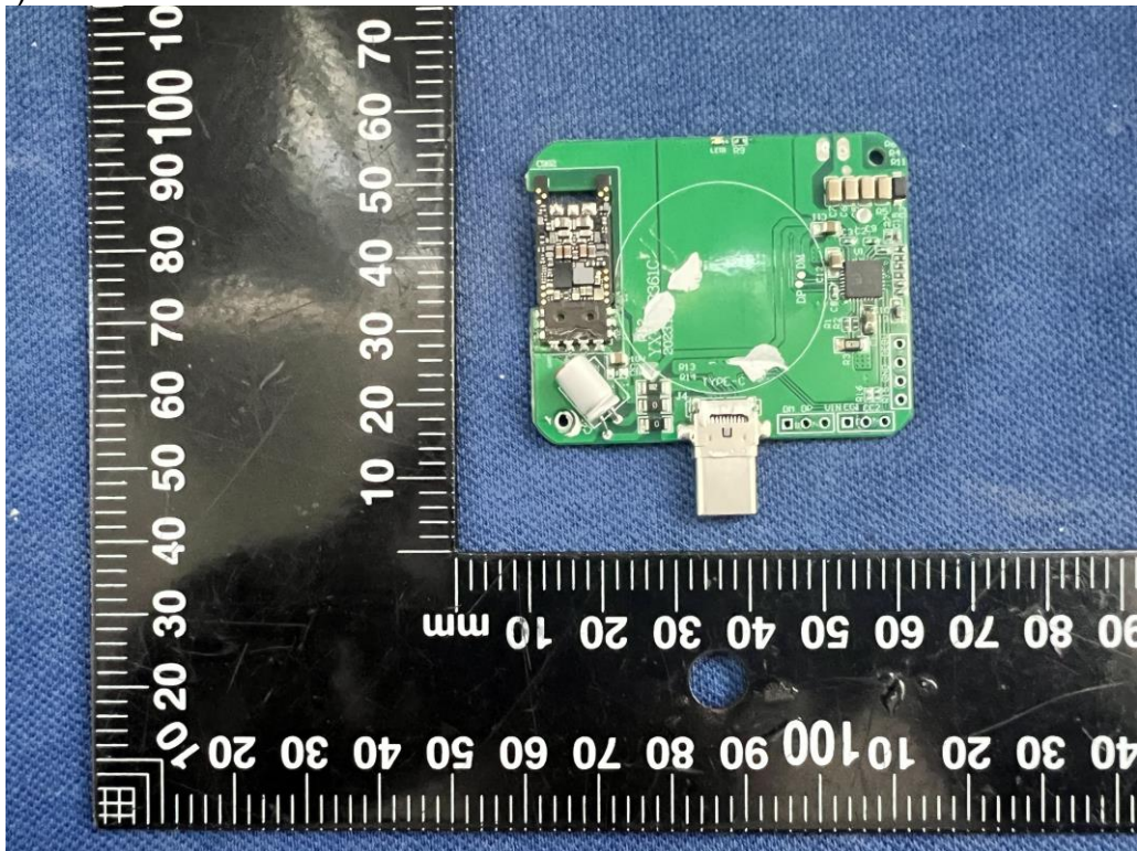
4) EUT Photo
