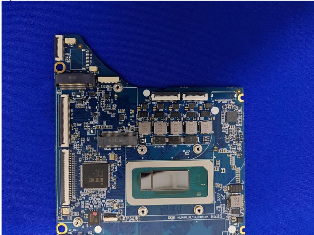
66) EUT Photo
