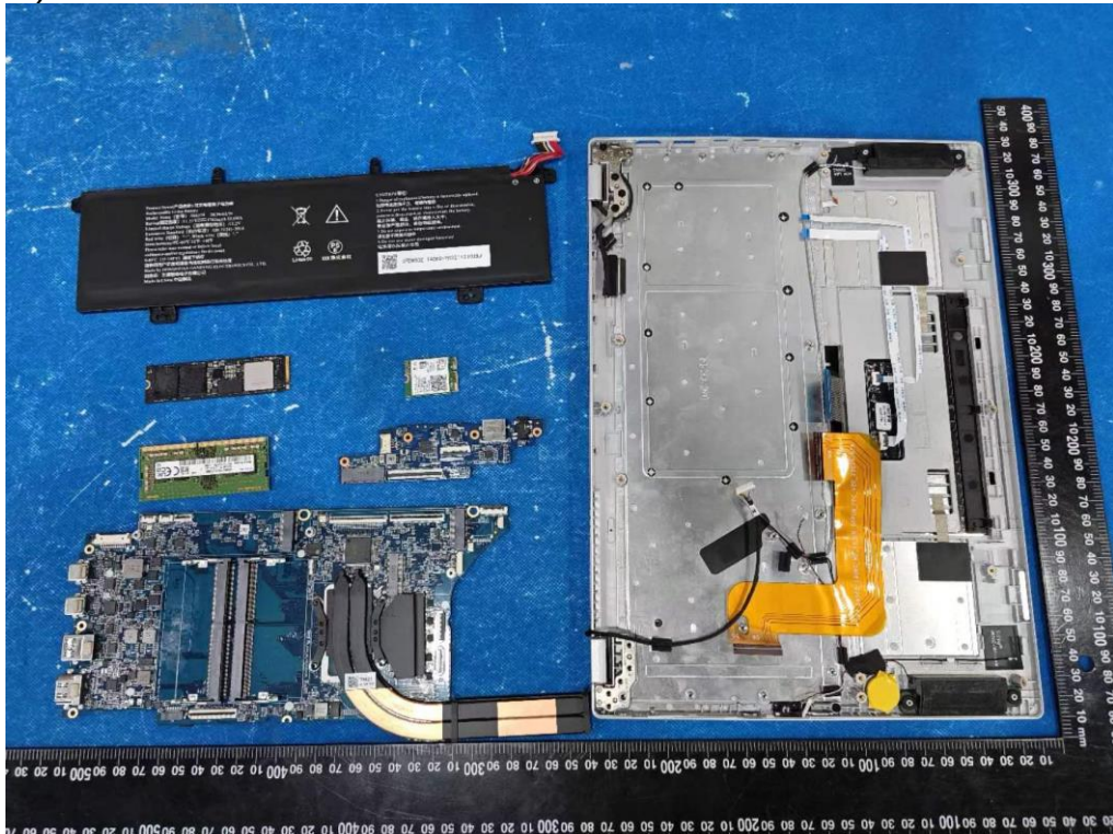
34) EUT Photo
