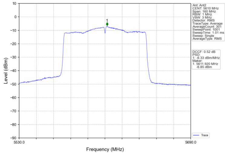
802.11ac(VHT80)_HCH_5610MHz_MIMO_NTNV
