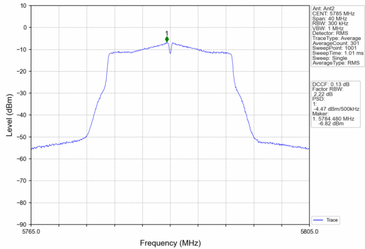
802.11n(HT20)_MCH_5785MHz_MIMO_NTNV
