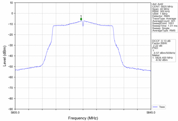
802.11n(HT20)_HCH_5825MHz_MIMO_NTNV
