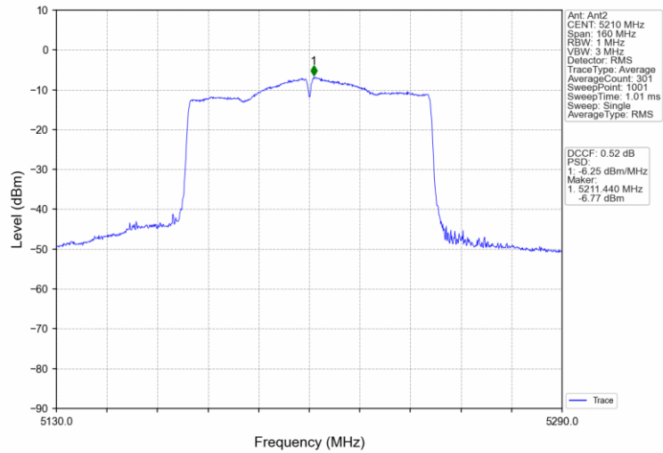
802.11ac(VHT80)_MCH_5210MHz_MIMO_NTNV
