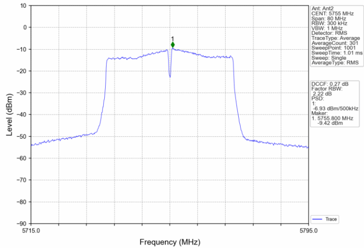
802.11n(HT40)_LCH_5755MHz_MIMO_NTNV
