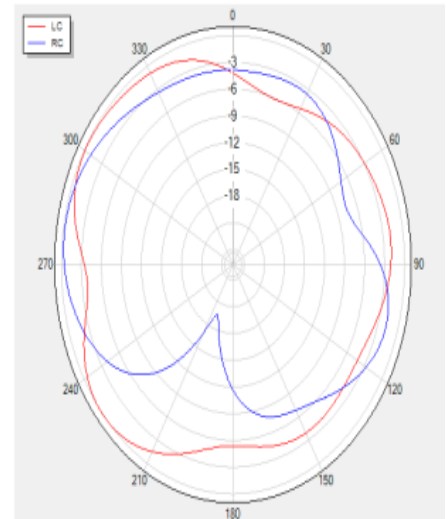
Theta=90 freq=2420MHz
