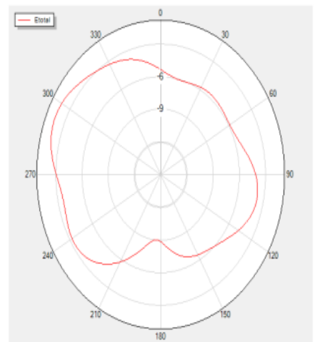
Theta=90 Freq=2420MHz
