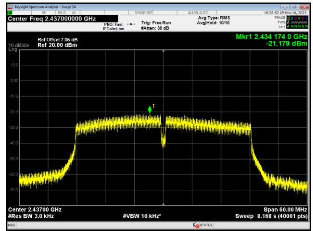
2437MHz
