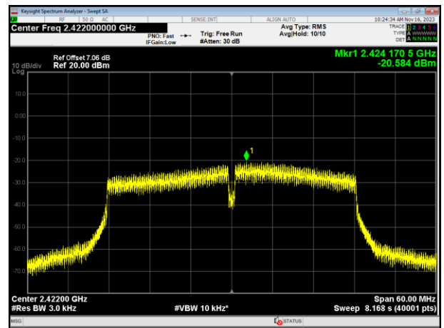
2422MHz
