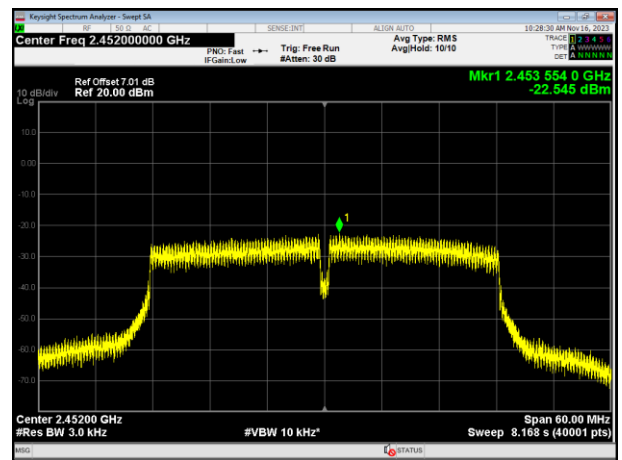
2452MHz
