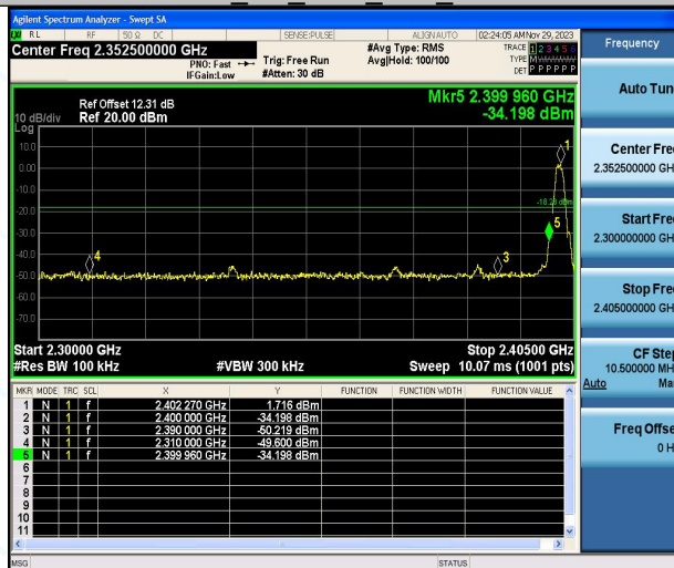
BLE_2M_Ant1_Low_2402
