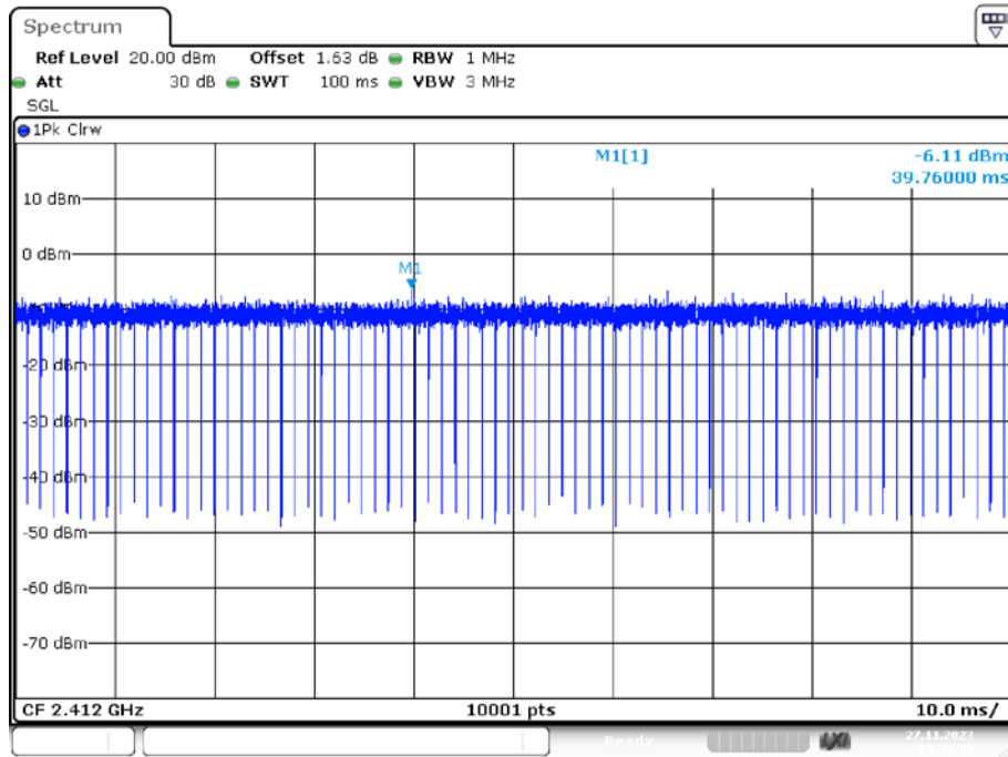
IEEE 802.11 n/HT20 2412MHz
