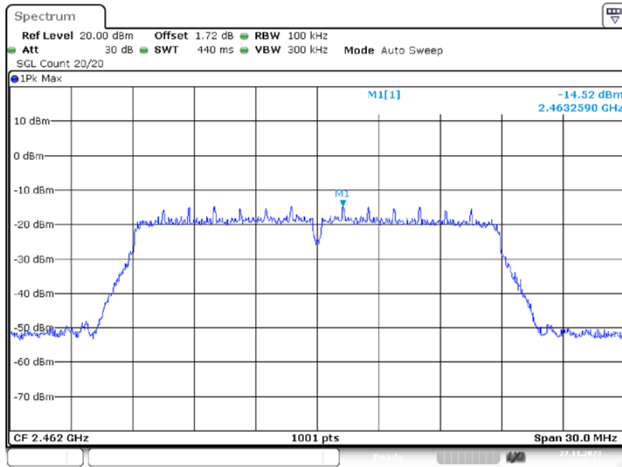
IEEE 802.11 n/HT20 2462MHz
