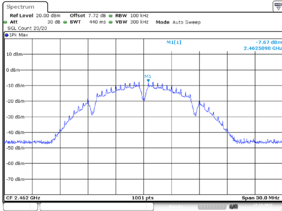
IEEE 802.11 b 2462MHz
