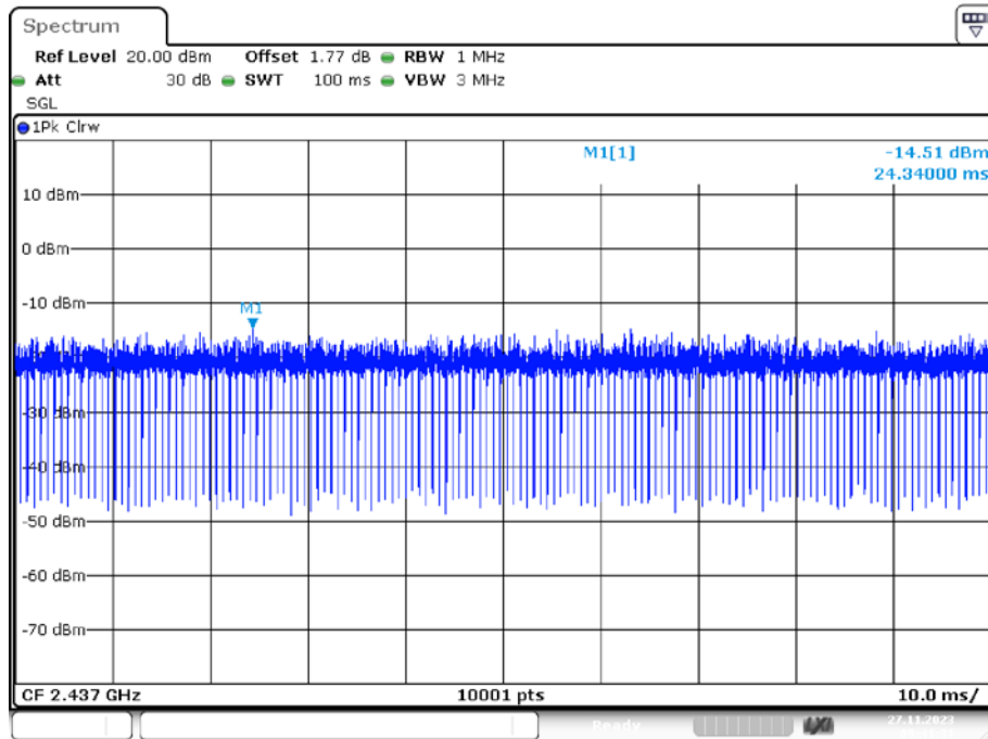
IEEE 802.11 n/HT40 2437MHz
