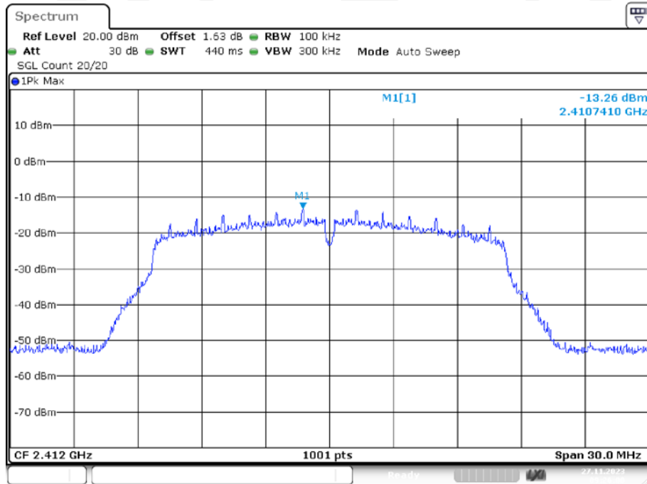
IEEE 802.11 g 2412MHz
