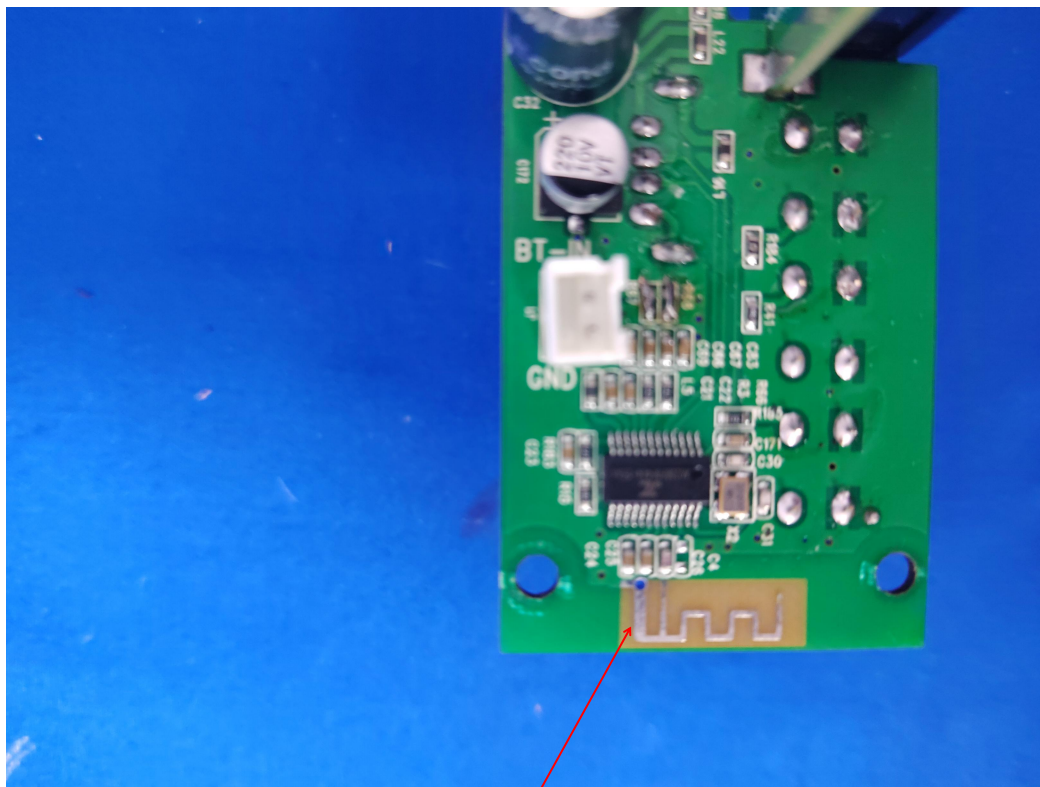
BT ANT
