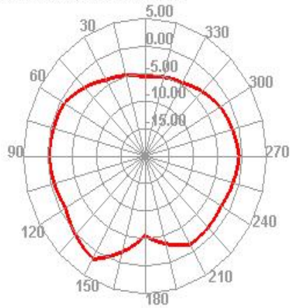
2400.000MHz E2
