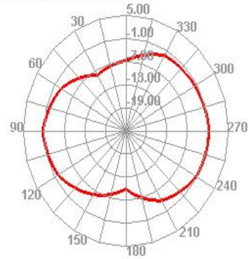
2450.000MHz H
