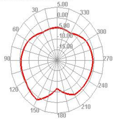
2450.000MHz E2
