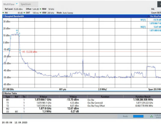
Band2-20MHz-QPSK-19100-6RB#0
