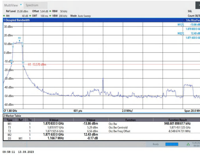
Band2-20MHz-16QAM-19100-5RB#0
