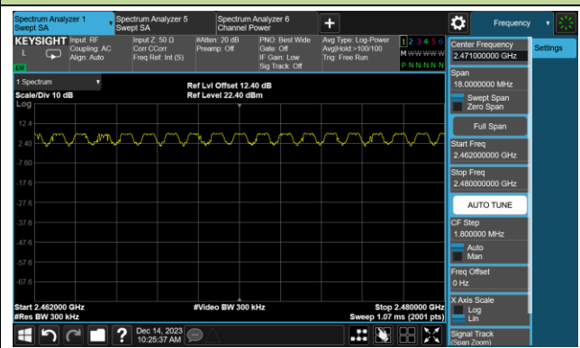
2462 ~ 2480MHz
