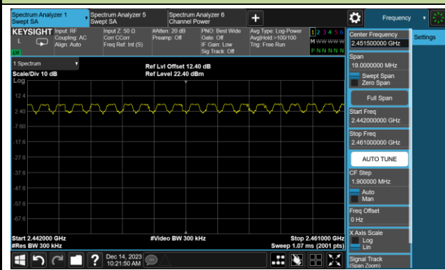
2442 ~ 2461MHz
