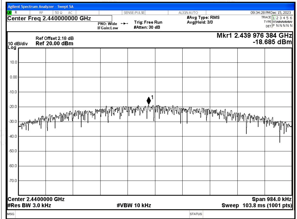
PSD NVNT BLE 2440MHz Ant
