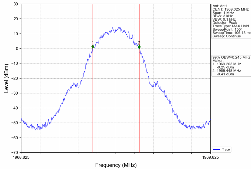
Band25_1969.325MHz_GMSK_SISO_Ant1_NTNV_Output_AGC+3
