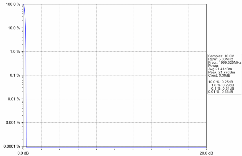
Band25_1969.325MHz_GMSK_SISO_Ant1_NTNV_AGC+3
