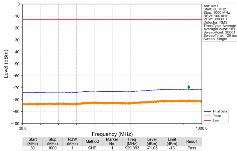
Band25_1932.5MHz_AWGN_SISO_Ant1_NTNV
