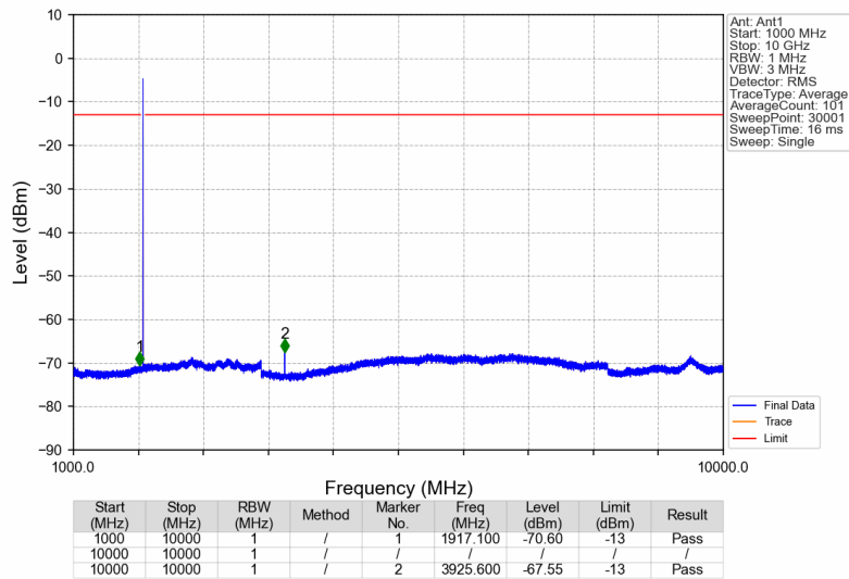
Band25_1962.5MHz_GMSK_SISO_Ant1_NTNV
