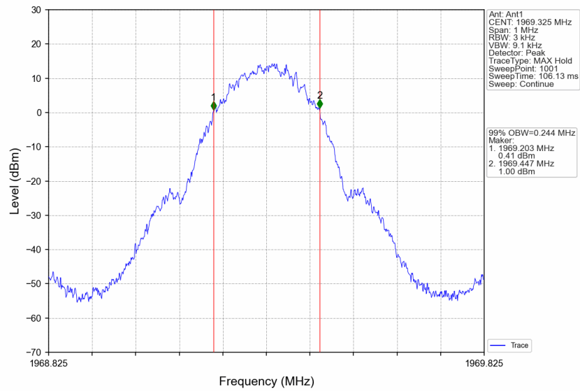
Band25_1969.325MHz_GMSK_SISO_Ant1_NTNV_Output_AGC+3
