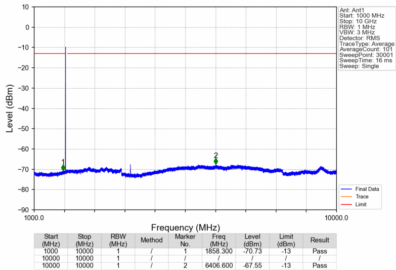
Band25_1932.5MHz_AWGN_SISO_Ant1_NTNV
