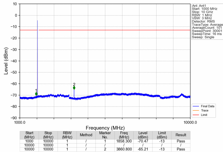
Band25_1930.1MHz_GMSK_SISO_Ant1_NTNV
