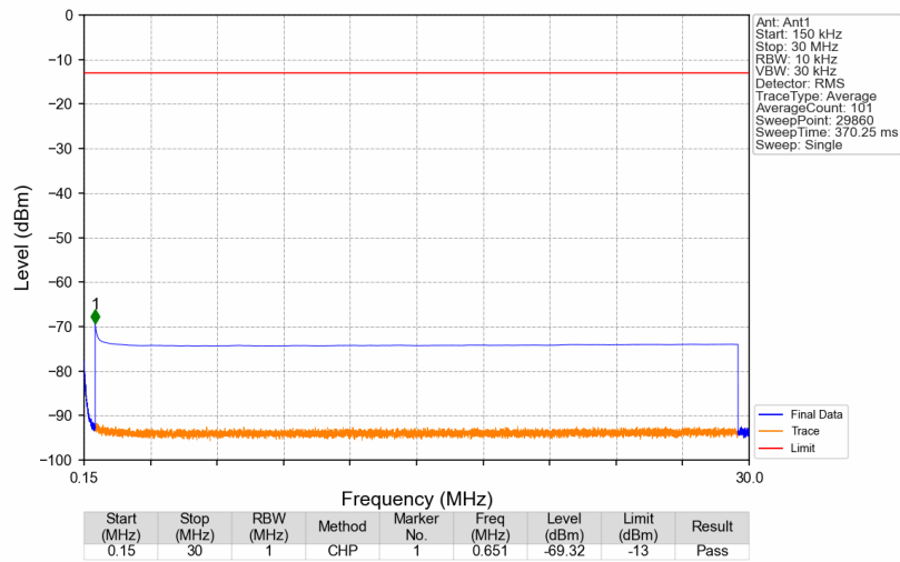
Band25_1994.9MHz_GMSK_SISO_Ant1_NTNV
