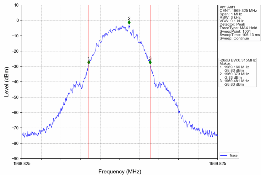
Band25_1969.325MHz_GMSK_SISO_Ant1_NTNV_Input_AGC+3
