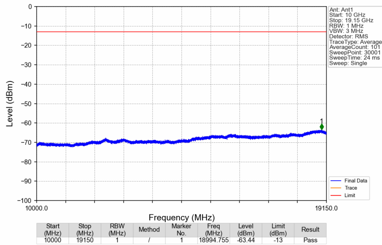
Band25_1932.5MHz_AWGN_SISO_Ant1_NTNV
