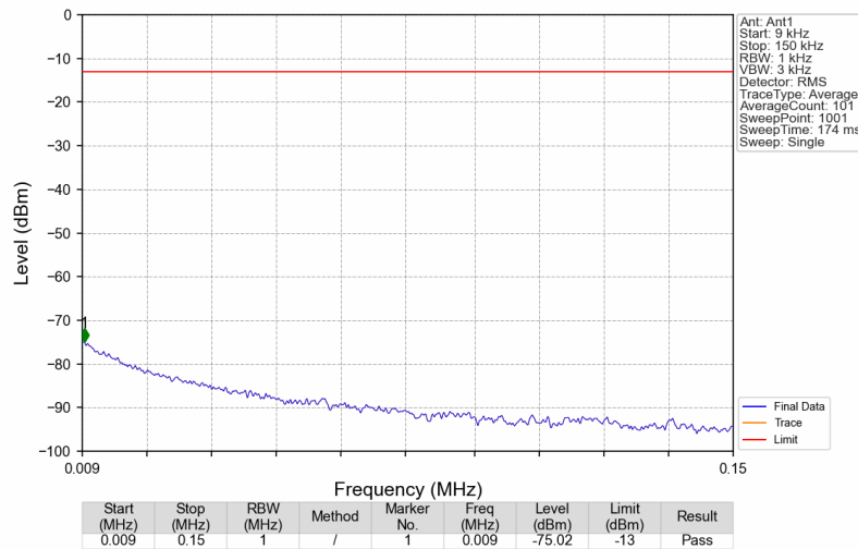
Band25_1962.5MHz_AWGN_SISO_Ant1_NTNV
