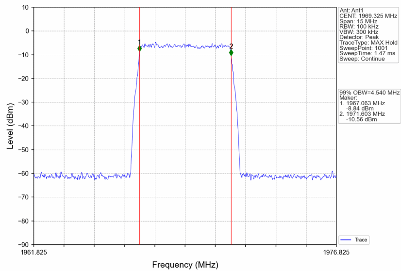
Band25_1969.325MHz_AWGN_SISO_Ant1_NTNV_Input_AGC+3
