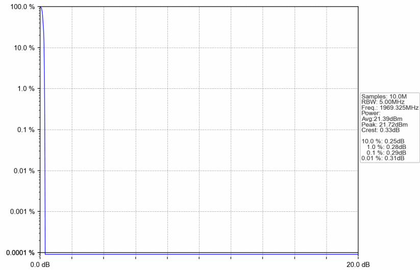
Band25_1969.325MHz_GMSK_SISO_Ant1_NTNV_AGC
