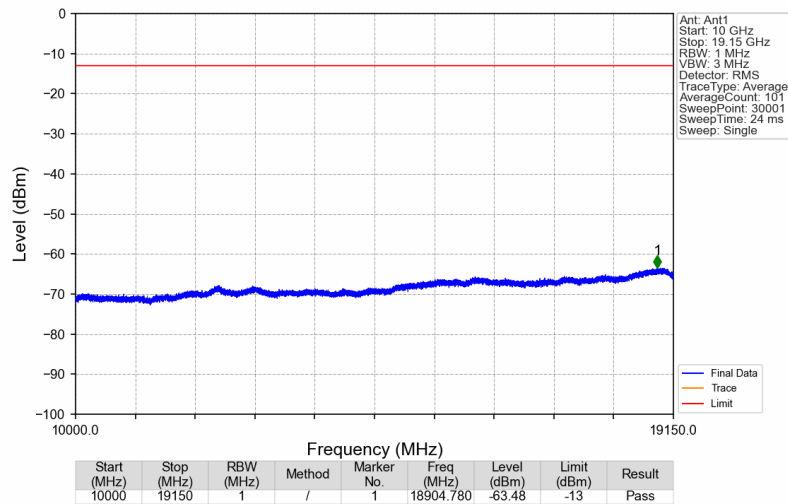
Band25_1930.1MHz_GMSK_SISO_Ant1_NTNV
