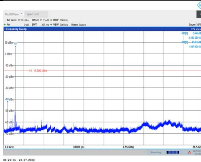
DH5_Ant1_2480_1000~26500
