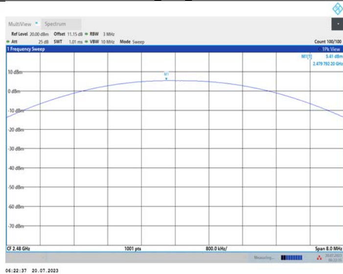
DH5_Ant1_2480
