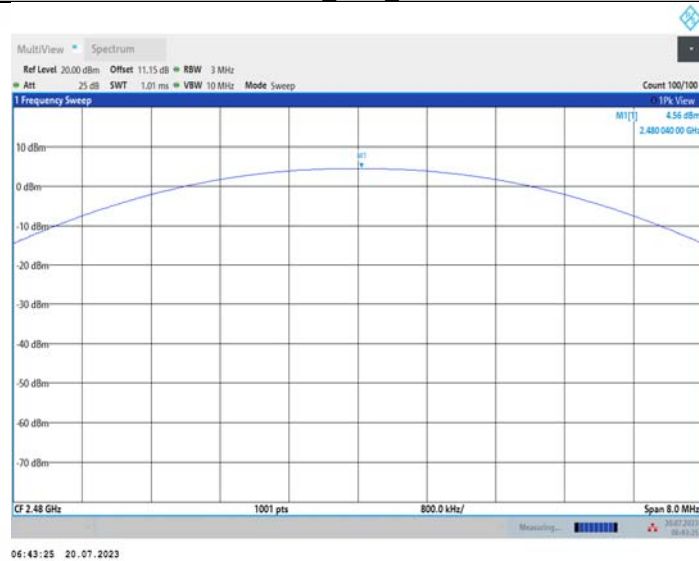
2DH5_Ant1_2480
