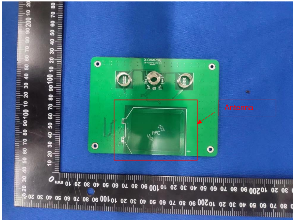
RF ID module
