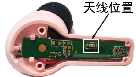
天线需放置在PCBA外层
