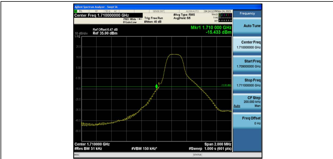
Band4-3MHz-QPSK-19965-1RB#14
