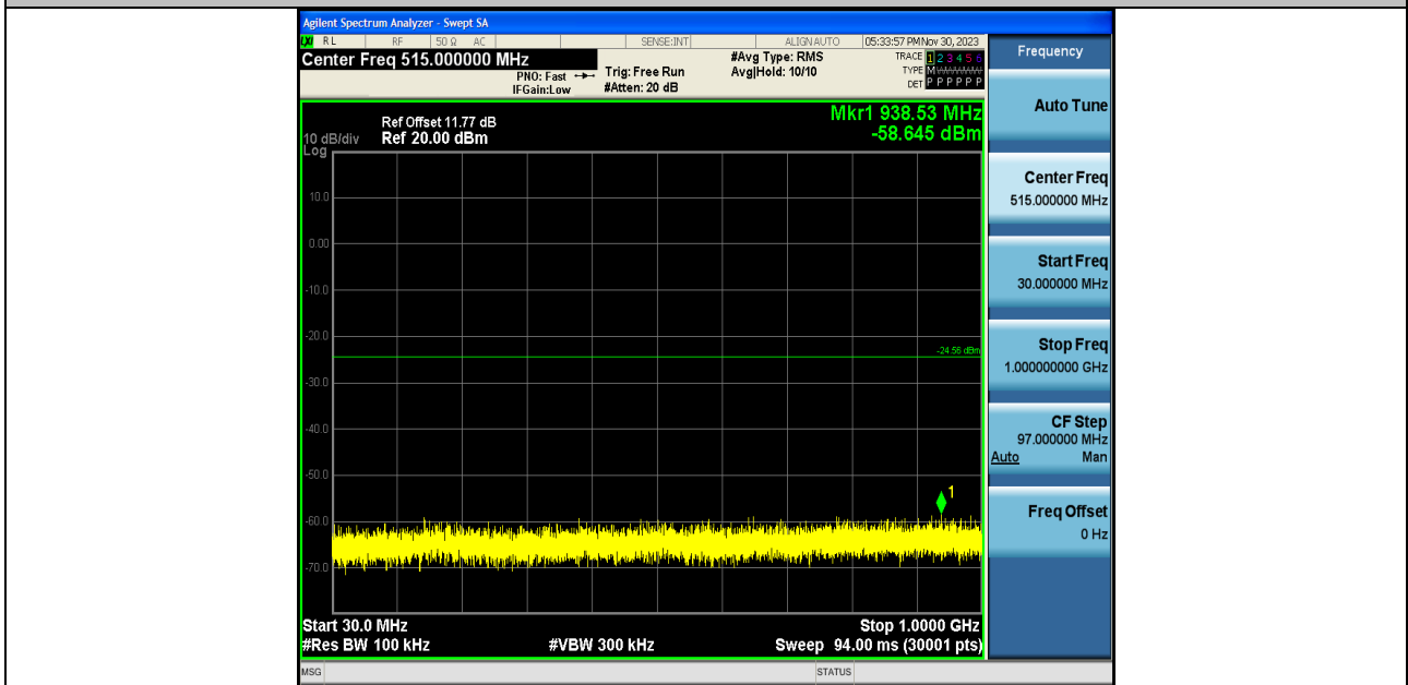
BLE_2M-Ant1-2440-30~1000-PASS
