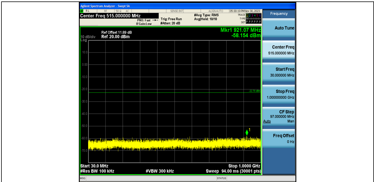
BLE_2M-Ant1-2404-30~1000-PASS
