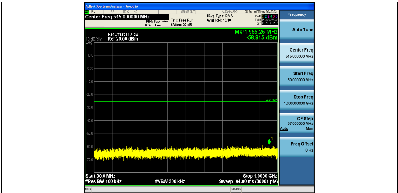
BLE_2M-Ant1-2478-30~1000-PASS
