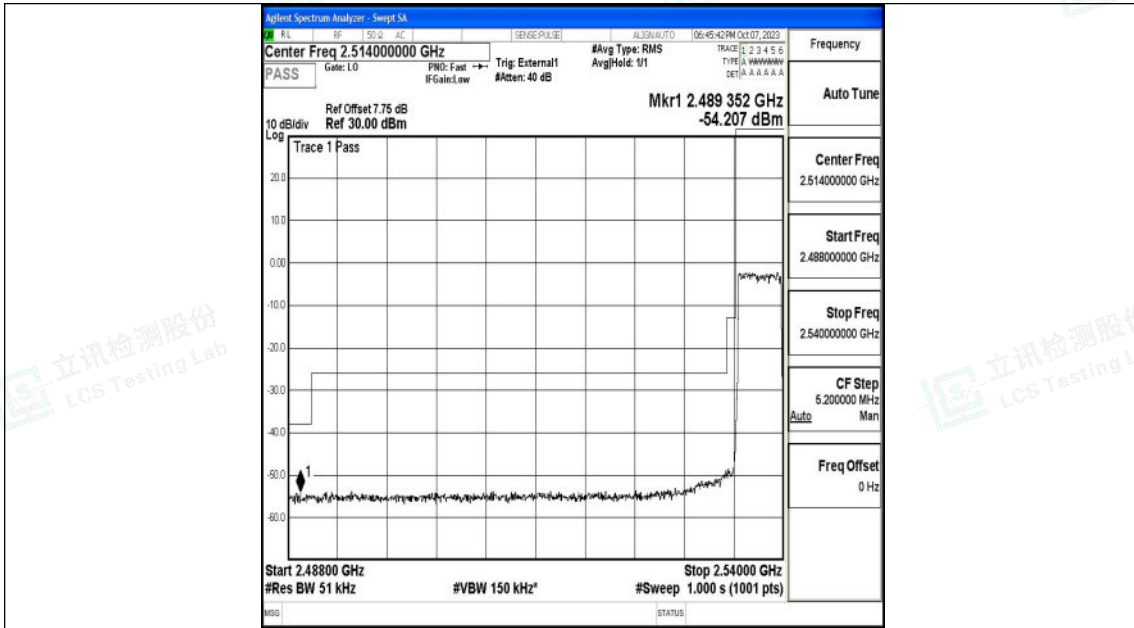
Band41_5MHz_QPSK_40065_25RB#0
