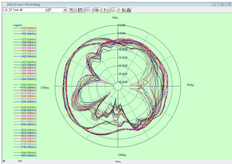
2.4GWIFI&Bluetooth&5G WIFI Phi=0deg
