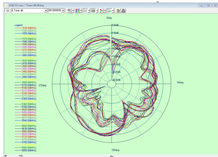
2.4GWIFI&Bluetooth&5G WIFI Theta=90deg
