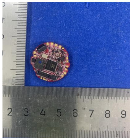
Antenna
