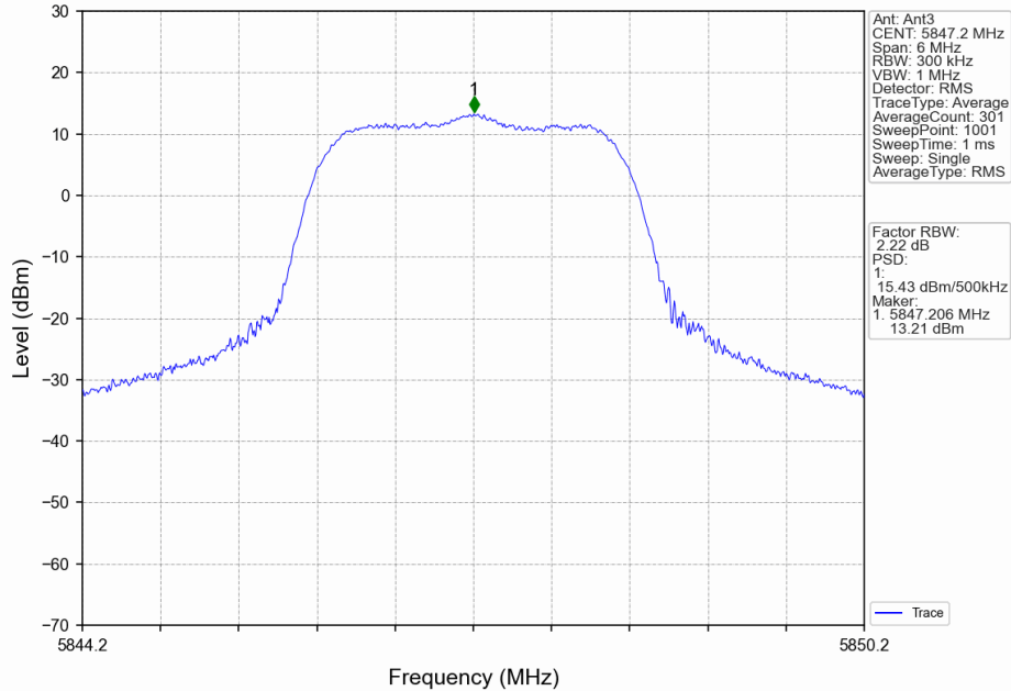
3M_HCH_5847.2MHz_MIMO_NTNV
