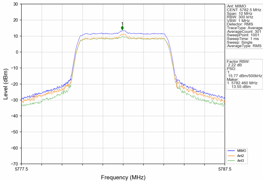
5M_MCH_5782.5MHz_MIMO_NTNV
