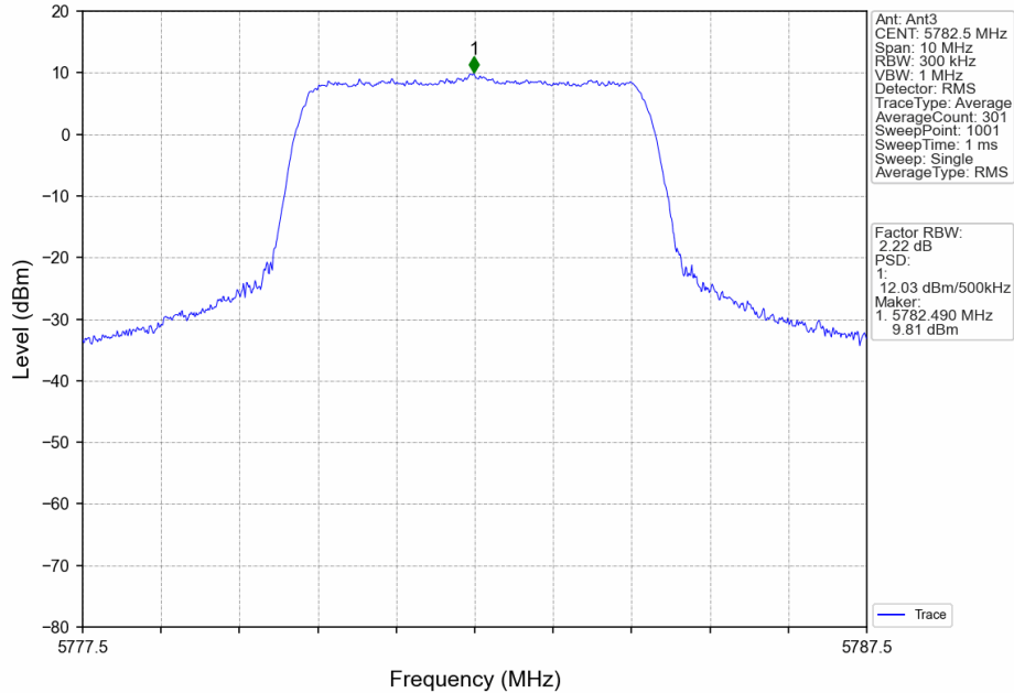
5M_MCH_5782.5MHz_MIMO_NTNV
