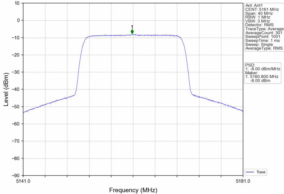
20M_LCH_5161MHz_MIMO_NTNV
