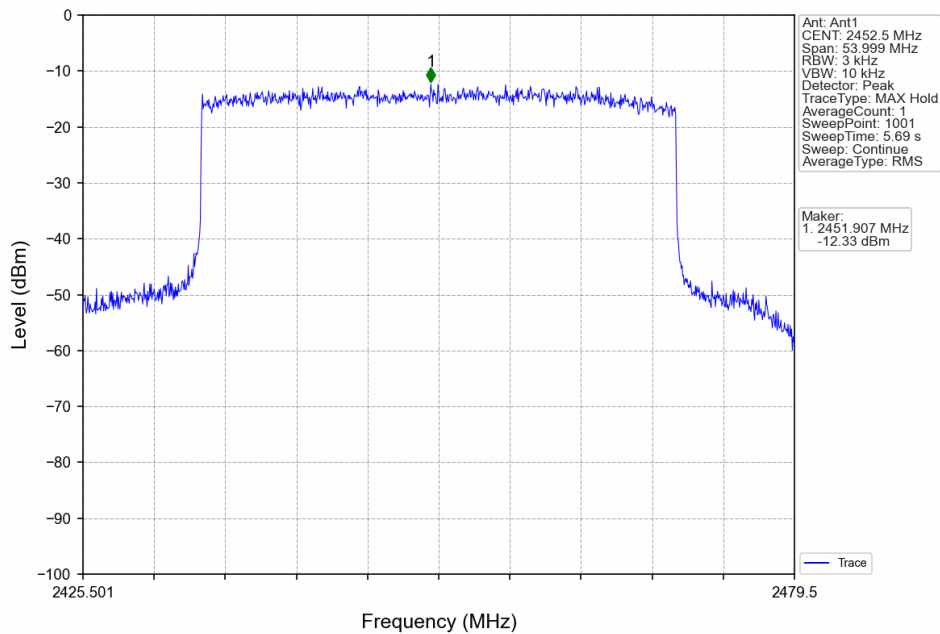
40M_HCH_2452.5MHz_MIMO_NTNV
