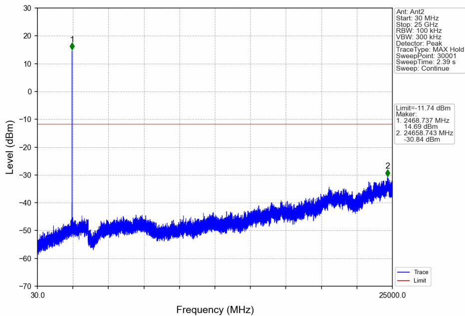
1.4M_HCH_2469.12MHz_Ant2_NTNV
