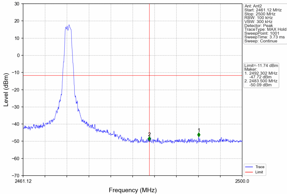
1.4M_HCH_2469.12MHz_Ant2_NTNV
