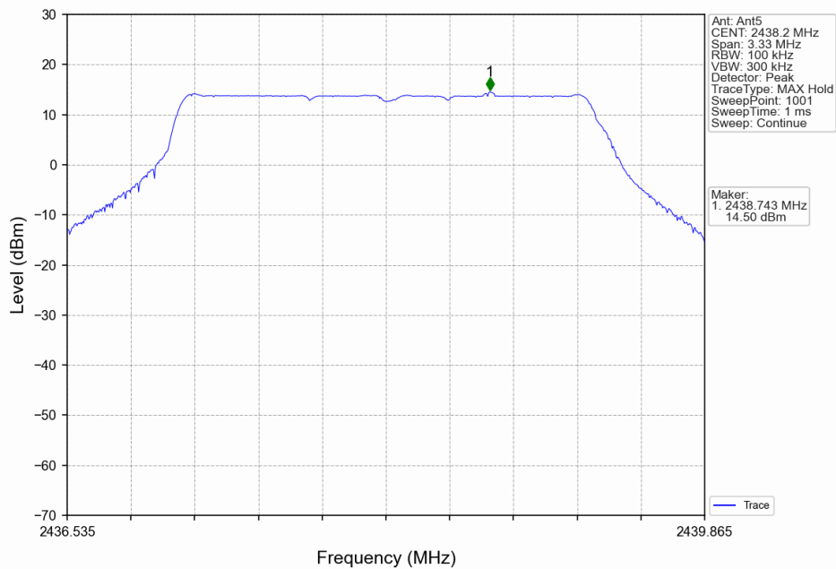
3M_MCH_2438.2MHz_Ant5_NTNV
