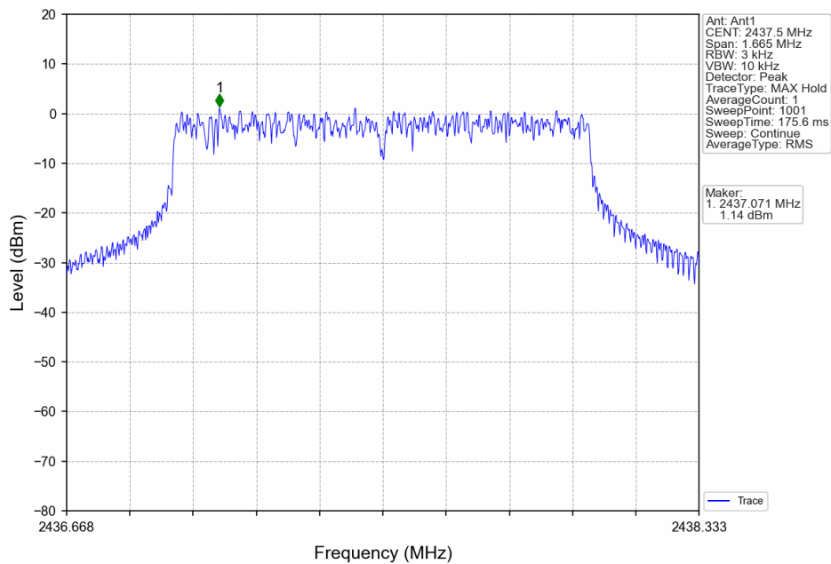
1.4M_MCH_2437.5MHz_Ant1_NTNV
