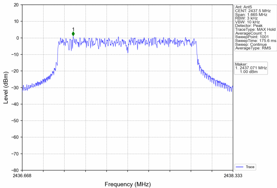
1.4M_MCH_2437.5MHz_Ant5_NTNV
