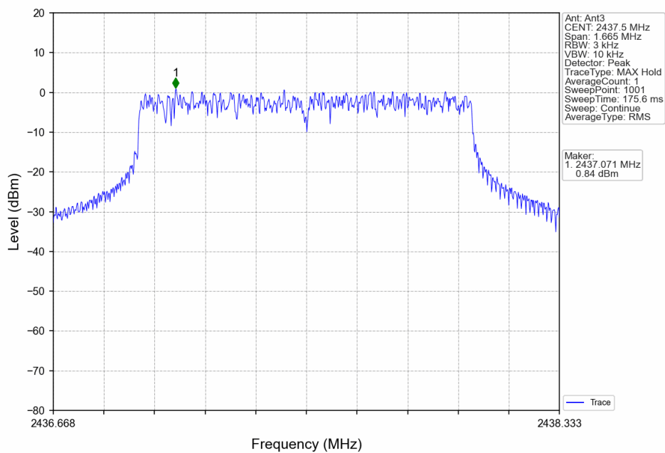
1.4M_MCH_2437.5MHz_Ant3_NTNV
